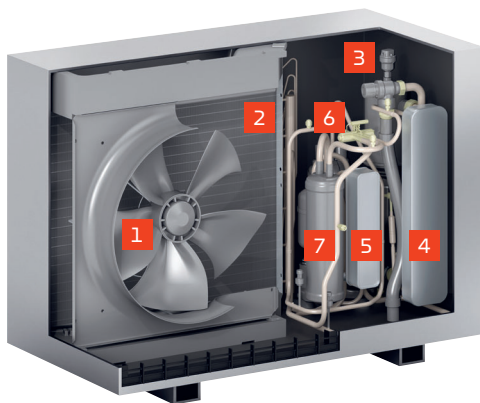
Außeneinheit ODU 150-A 2,1 bis 8,0 kW (A7/W35)
