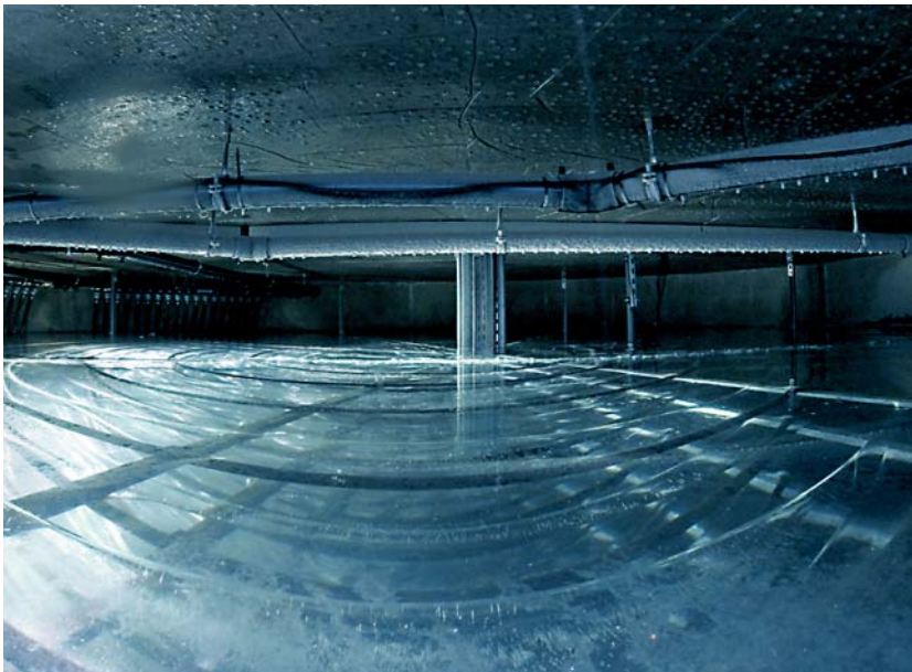
Die Kristallisationsprozesse im Eisspeicher können per Kameraübertragung visualisiert werden.
