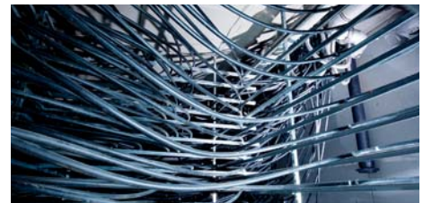
Das Leitungssystem des Eisspeichers ist in einer 18 mal 25 Meter großen Betonzisterne verbaut.
