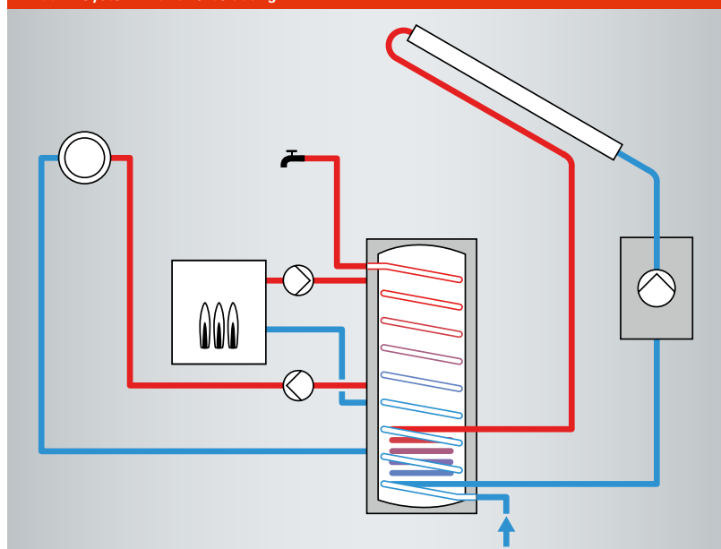
Abb. 7 System mit Pufferbeladung
