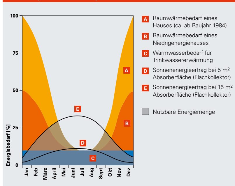
Abb. 1 Energiebedarf und Solarertrag
