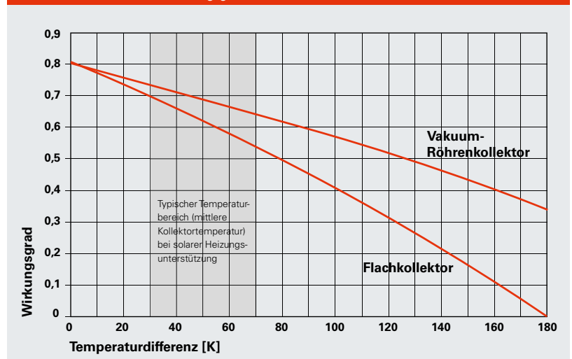
Abb. 3 Charakteristische Wirkungsgradkurven
