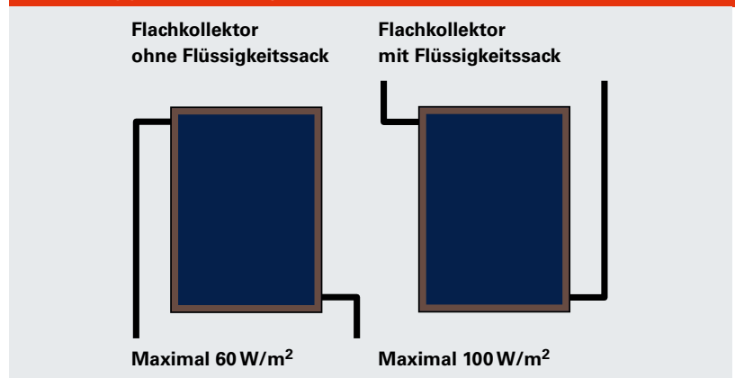
Abb. 2 Dampfproduktionsleistungen von Kollektoren
