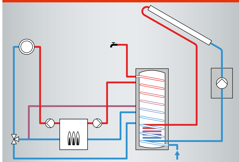
Abb. 6 System mit Rücklaufanhebung
