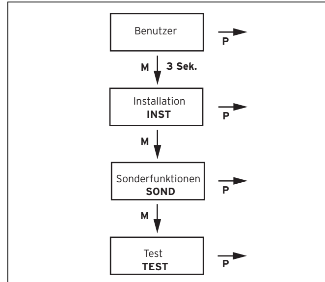
Abb. 4.1 Menüstruktur
