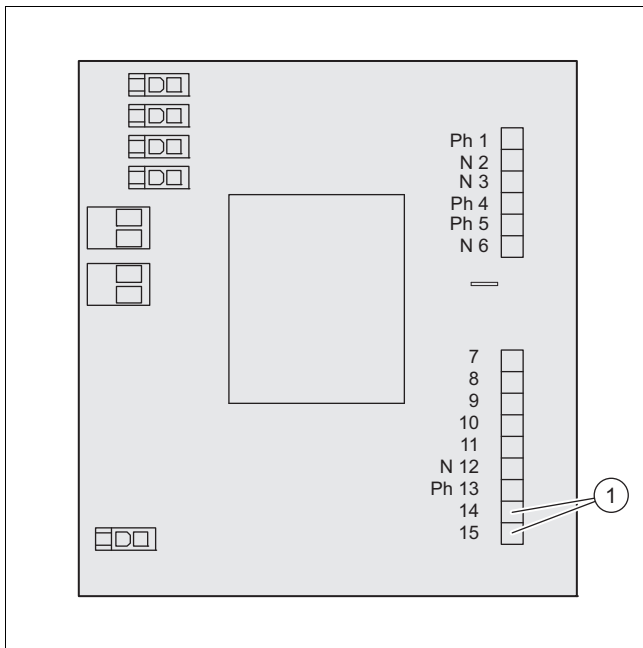
1 Salida 14-15
