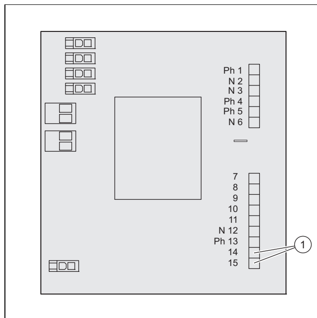
1 Uitgang 14-15
