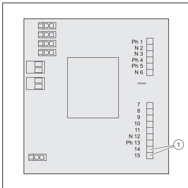
1 Saída 14-15
