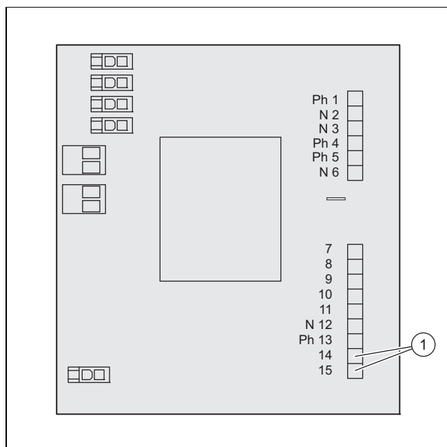
1 Uscita 14-15
