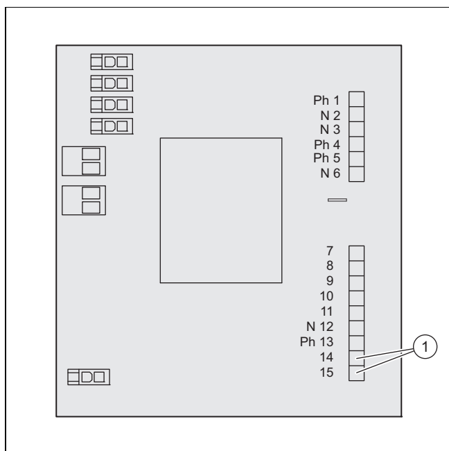
1 Utgang 14–15
