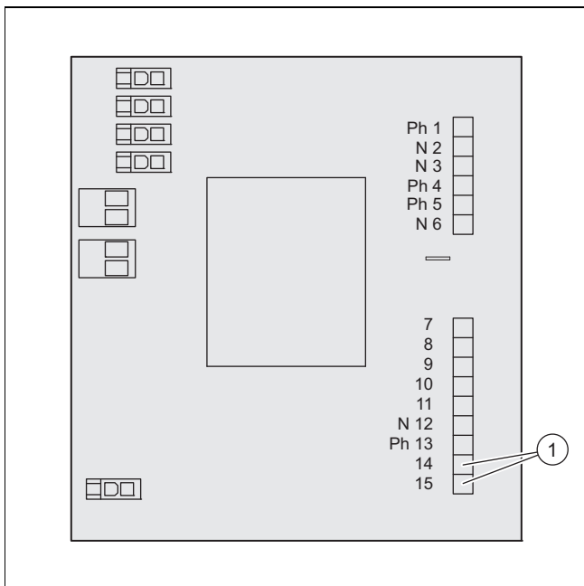
1 Izlaz 14-15
