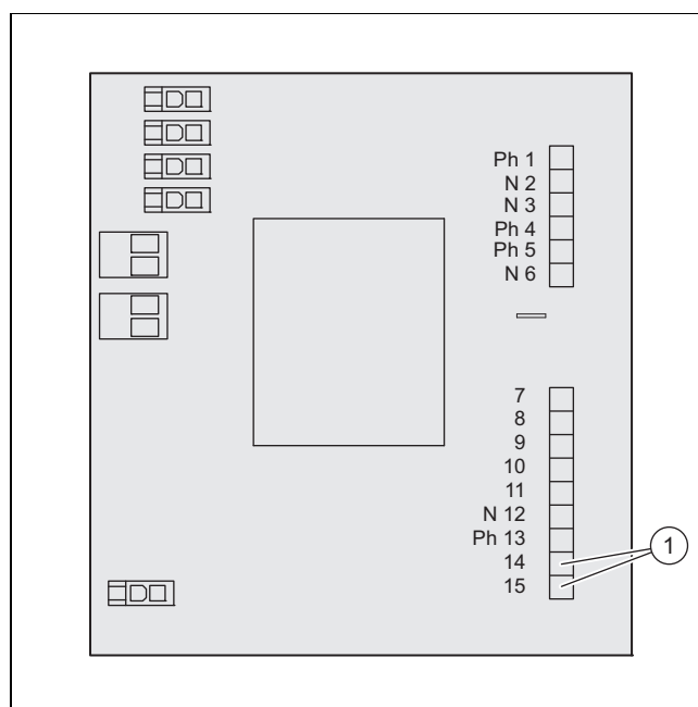
1 Izlaz 14-15
