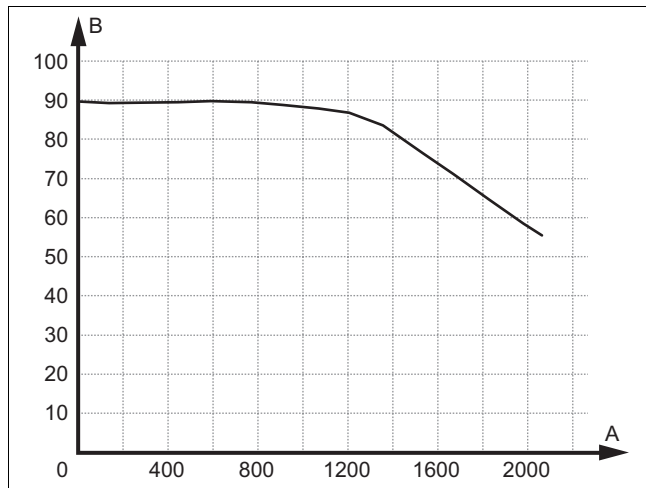
A Portata volumetrica, in l/h B Pressione di mandata residua, in kPa
