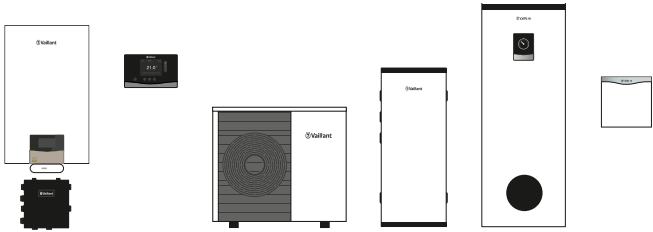
ecoTEC exclusive VC mit Internetmodul, Hybrid-Kit, sensoCOMFORT 720, aroTHERM plus, Pufferspeicher VR RW 45/2B, uniSTOR exclusive VIH R, VR 71
