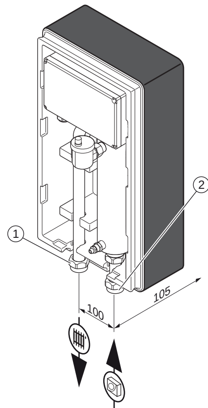
1 Vorlauf Anlage 1"
