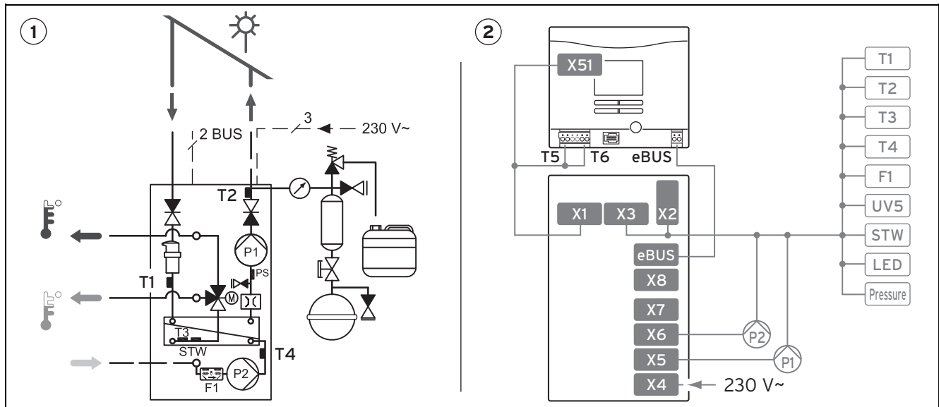
1 Hydraulikschema
