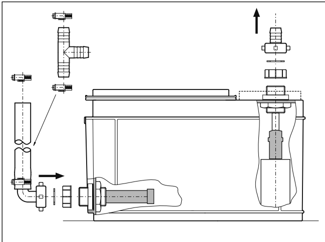
4.2 Neutralisationseinrichtung mit Förderpumpe montieren
