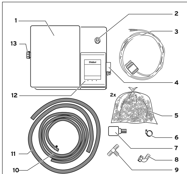
4.1 Übersicht der Neutralisationseinrichtung mit Förderpumpe
