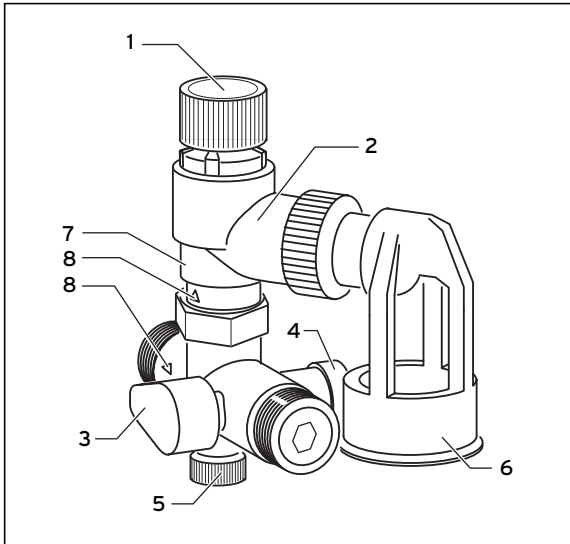
Abb. 3.1 Sicherheitsgruppe
