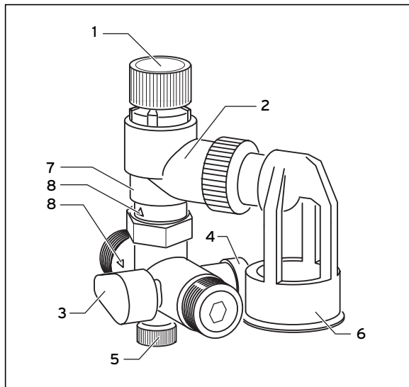
Рис. 3.1 Система безопасности
