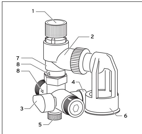
3.1 ábra Biztonsági szerelvényecsoport
