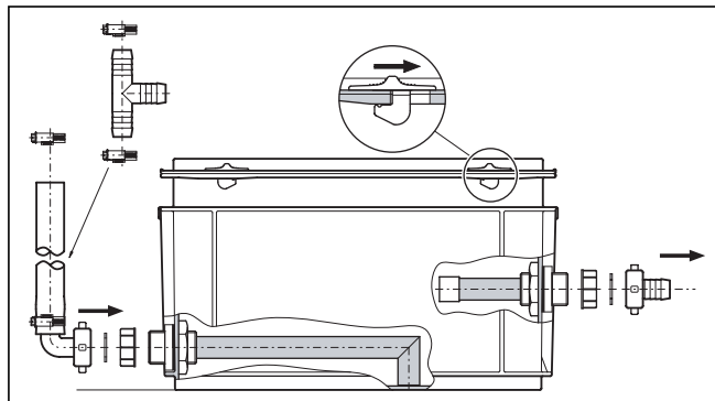
Sl. 3.4 Priključak naprave za neutralizaciju bez pumpe za napajanje
