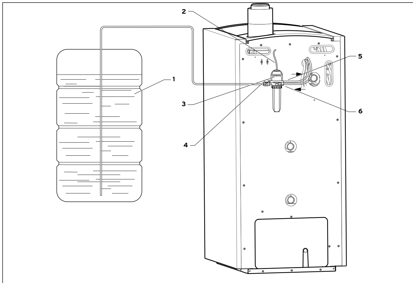
Abb. 4.1 Einbaubeispiel Heizöhlüfter
