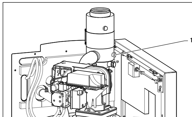
Abb. 5.1 Entgasungsleitung an icoVIT installieren
