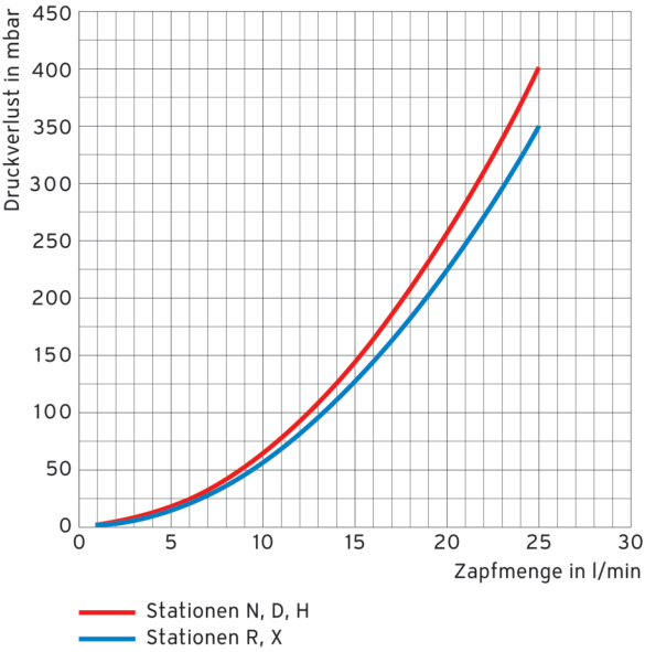
Druckverluste sekundär
