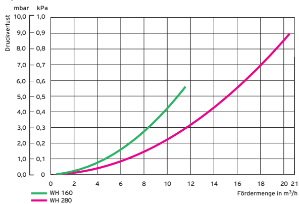
Hydraulische Weiche WH 160 und WH 280
