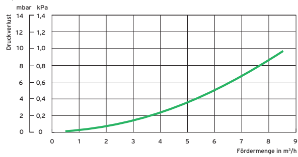
Hydraulische Weiche WH 95
