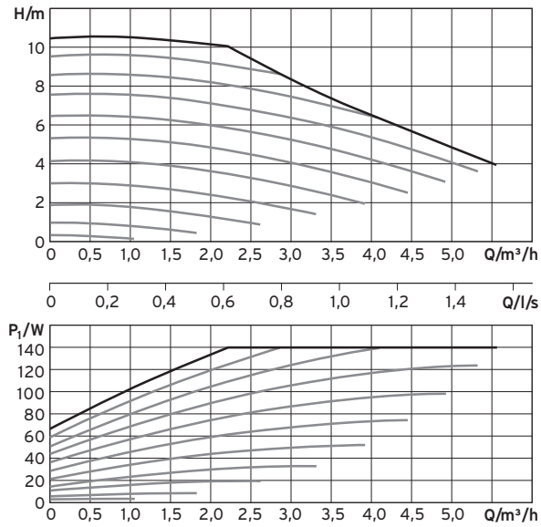
Druckverlustdiagramm Grundfos Pumpe UPML 25-105
