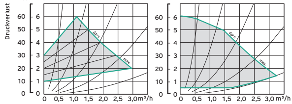
Druckverlustdiagramm Rohrgruppen 0020191813,14,17,788 mbar kPa
