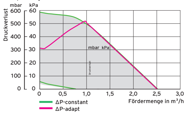
Pumpendiagramm Einbau-Sets eco/auroCOMPACT
