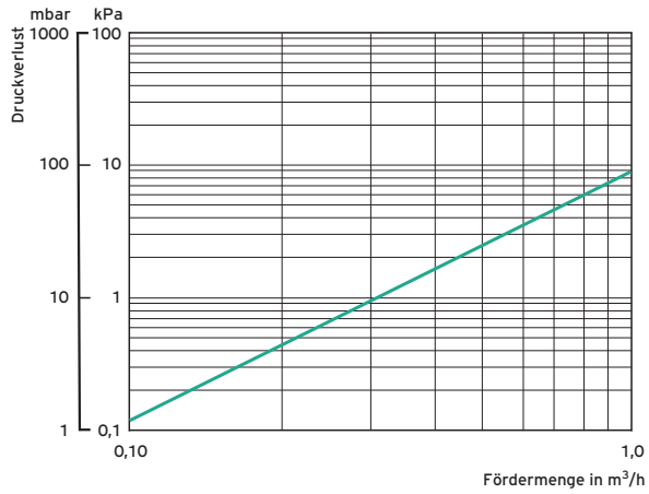
Verteilerbalken WHV 35
