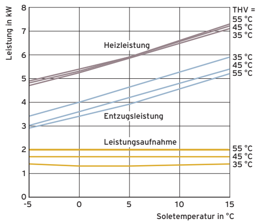
Leistungsdiagramm VWF 57/4
