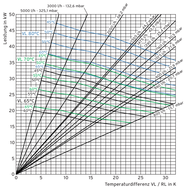
Leistungdiagramm VIH R 300
