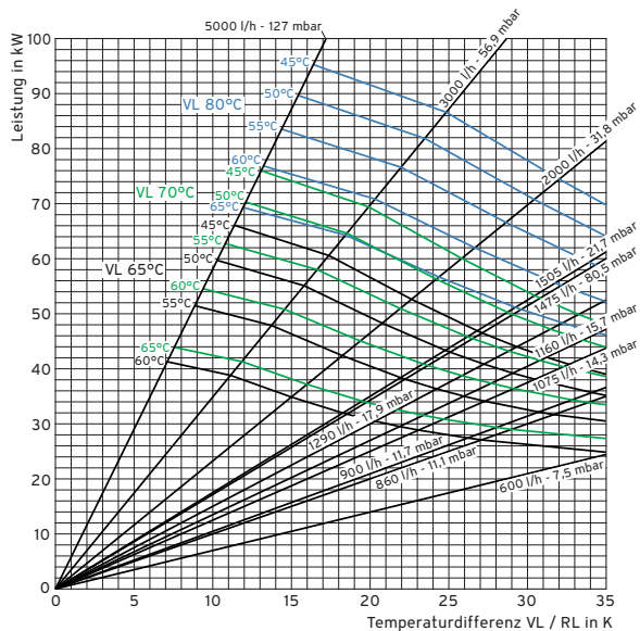
Leistungdiagramm VIH SW 400
