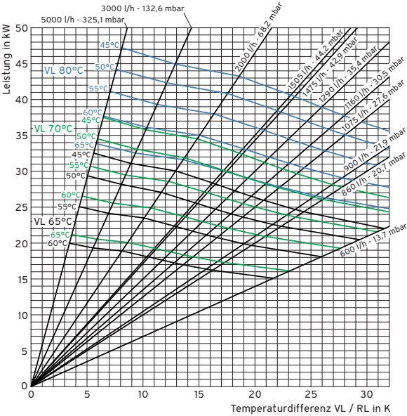
Leistungsdiagramm VIH R 300
