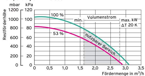
Pumpendiagramm VC 656
