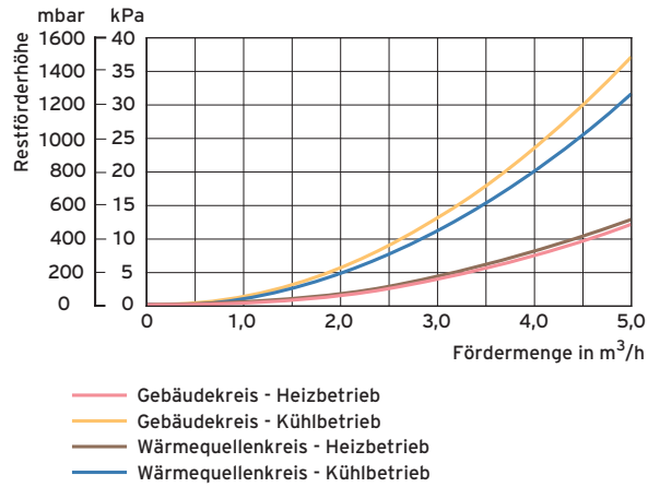
Druckverlustdiagramm VWZ NC 19
