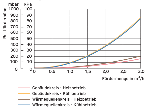
Druckverlustdiagramm VWZ NC 11
