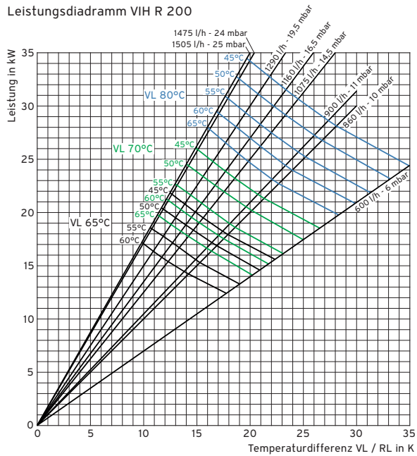
Leistungsdigramm VIH R 200
