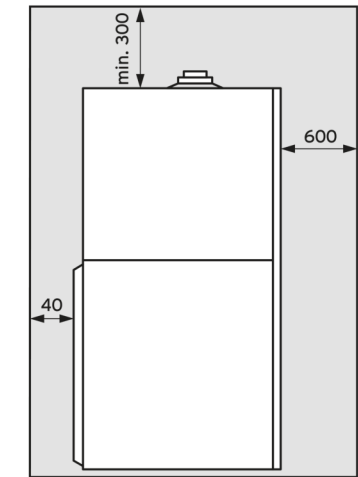
Seitenansicht
