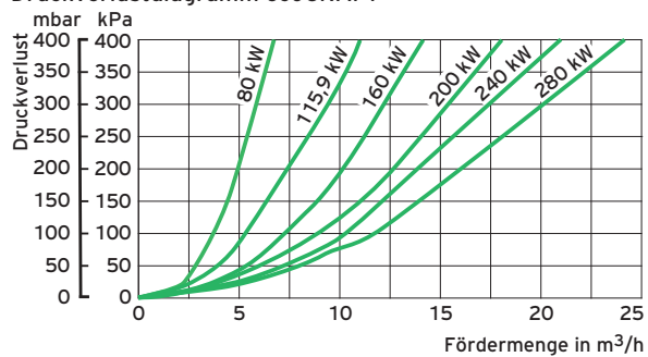
Druckverlustdiagramm ecoCRAFT
