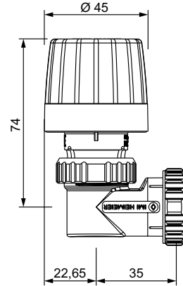
Winkelanschluss mit EMOtec
