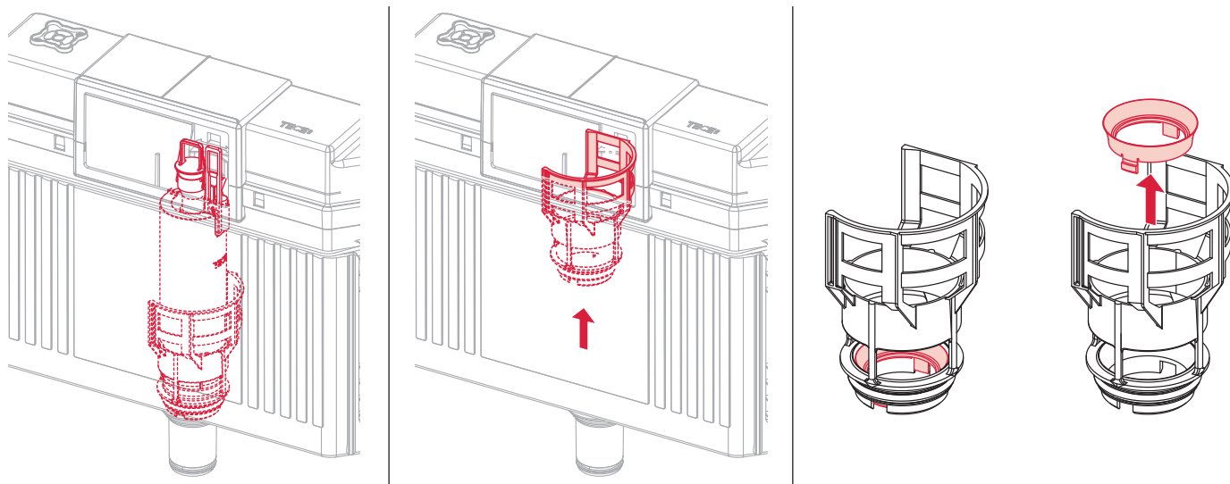
9820337 – Drosselset / Throttle set / Jeu de bague de réglage de débit / Set di riduzione pressione / Set de estrangulamiento / Zestaw dławika / Комплект ограничительных
