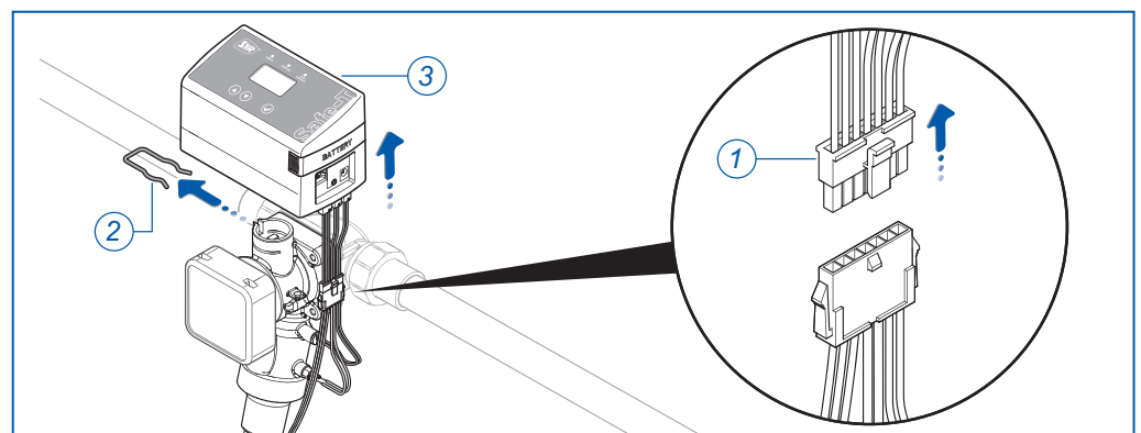
Abb. 9: Steuerung demontieren
