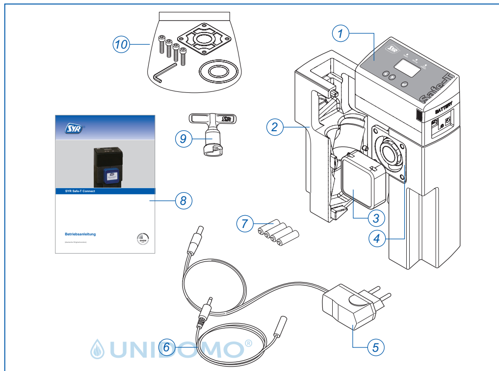
Abb. 1: Lieferumfang SYR-Safe-T Connect
