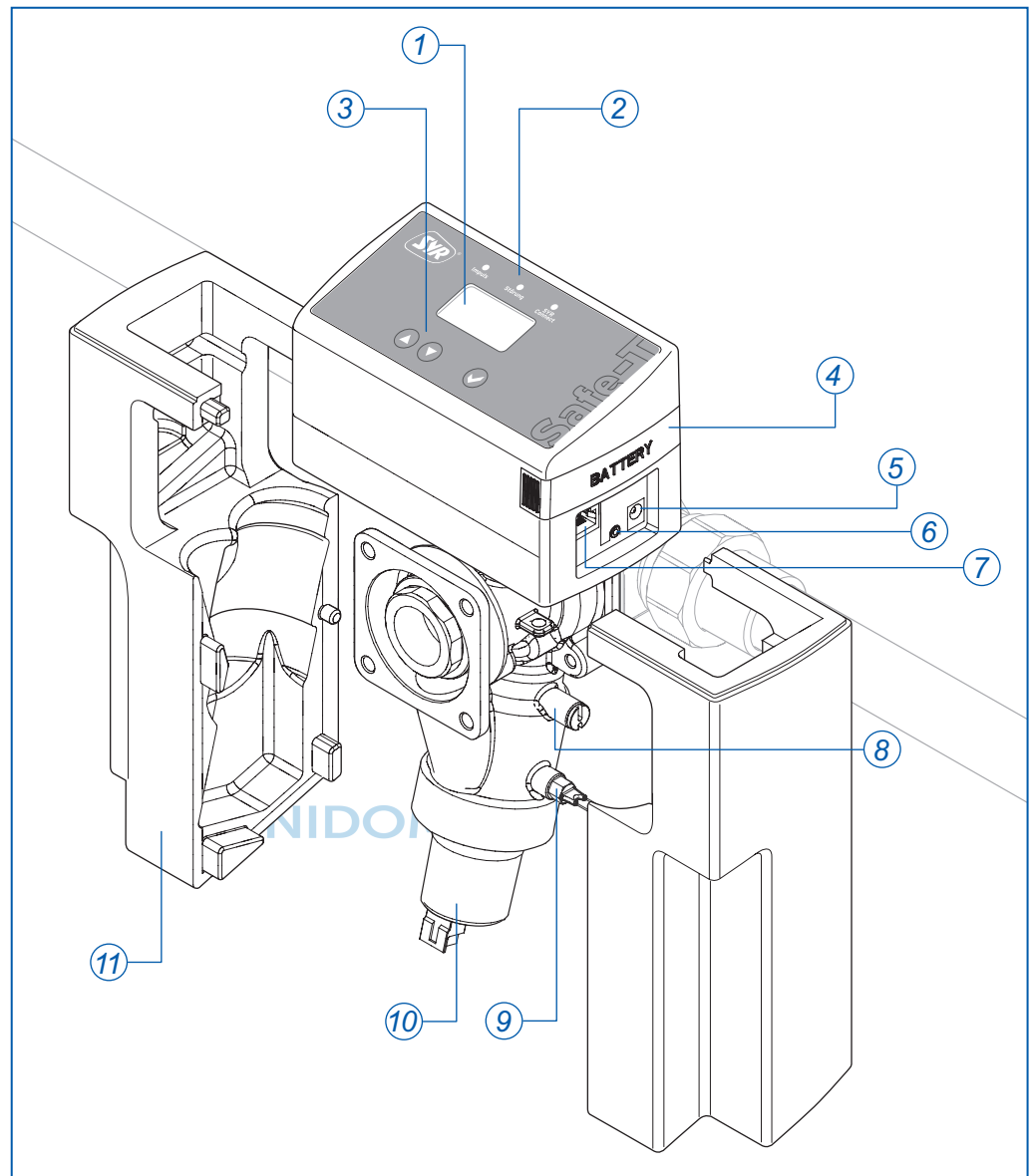
Abb. 2: Aufbau SYR-Safe-T Connect
