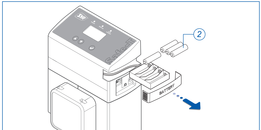
Abb. 4: Batterien einlegen
