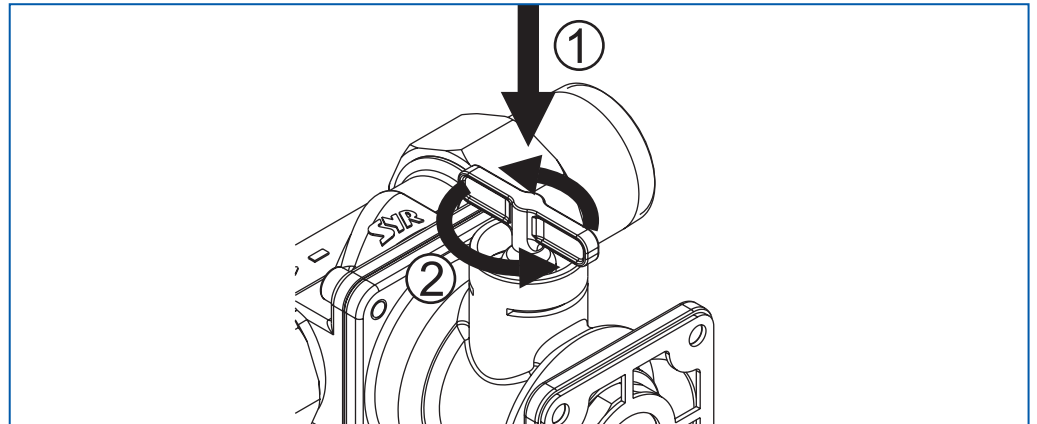
Abb. 10: Absperrung öffnen
