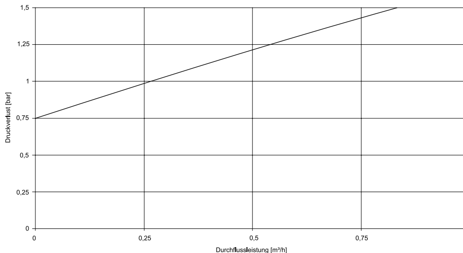
Leistungsdiagramm BA FüllCombi Plus 6628 mit Wasserzähler
