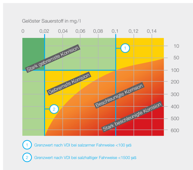
Korrosionsverhalten in Abhängigkeit von Leitfähigkeit und Sauerstoff
