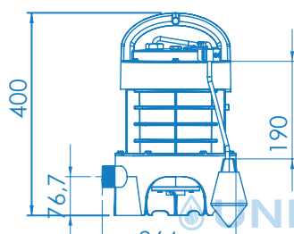
SANIPUMP® mit Zerkleinerungsschneidwerk
