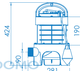
SANIPUMP® Vortex
