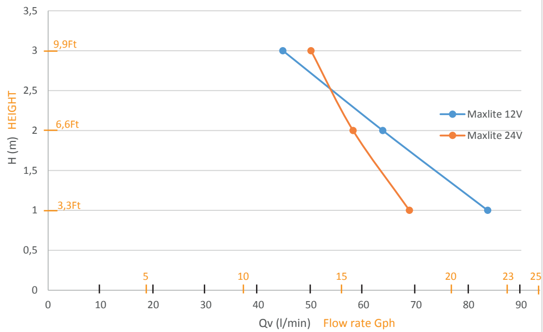
Performance Maxlite 12V et 24V
