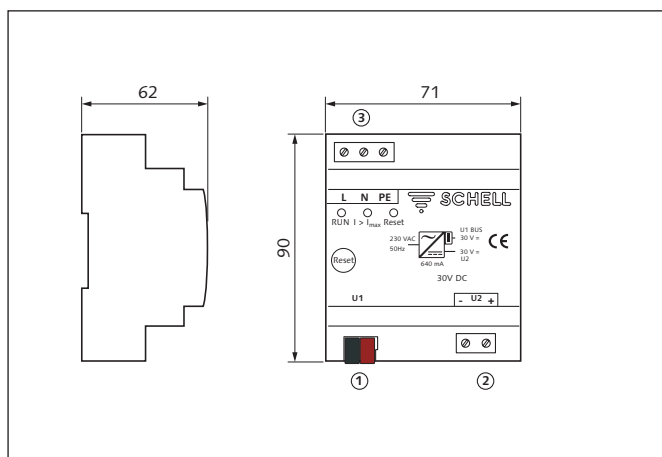
Plan coté – Bloc d'alimentation eSCHELL
