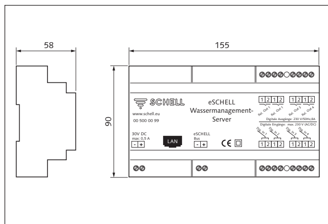
Plan coté – Serveur de gestion d'eau eSCHELL
