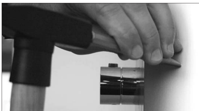
3. Bohrlöcher kornen.
