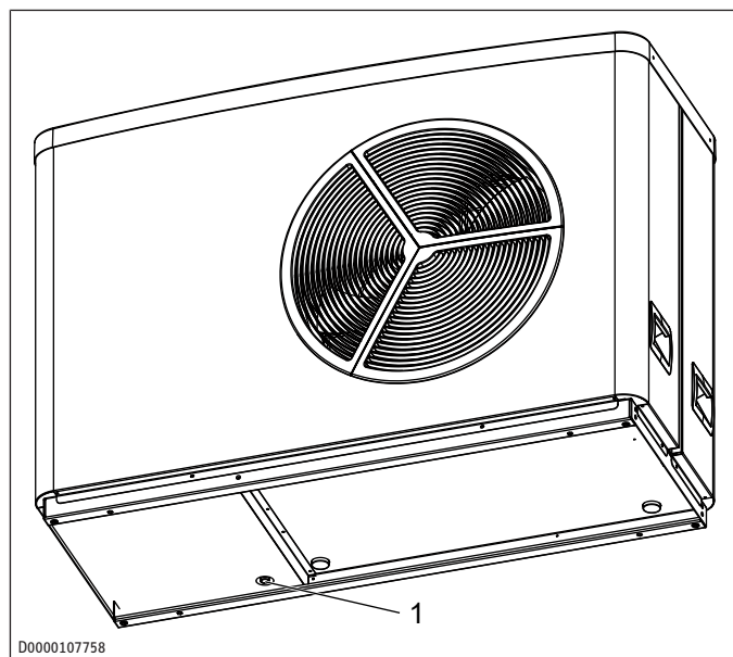
1 Kondensatablauf
