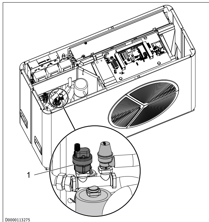
1 Entlüftungsventil
