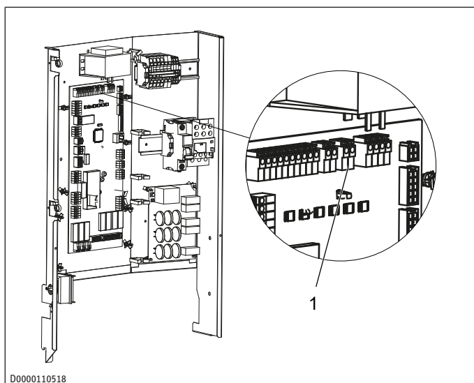
1 T35: Anschluss Außen-temperaturfühler
