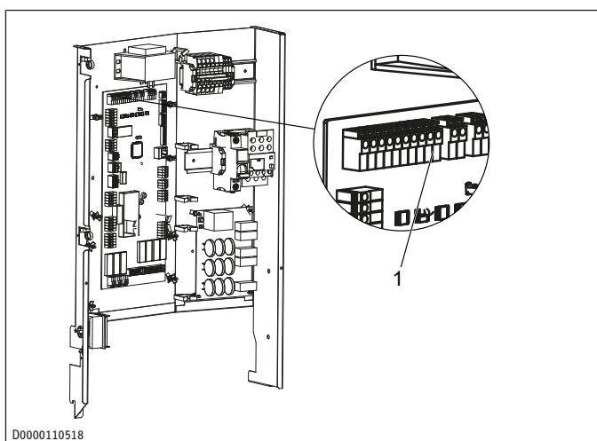
1 T33: Anschluss Anlege-fühler
