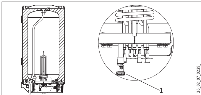
1 Kap aftapkraan
