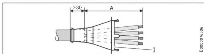
1 Kabeltule
