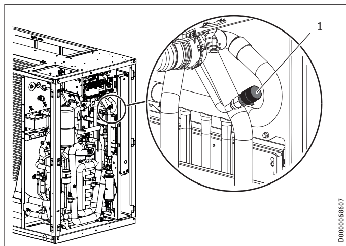
1 Entlüftungsventil
