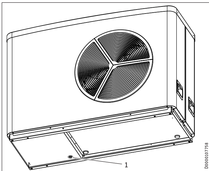
1 Kondensatablauf
