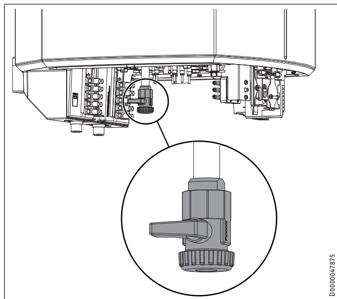
1 Entleerungsventil mit Schlauchanschluss G 3/4
