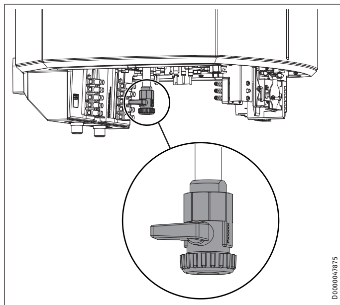
1 Vypúšťací ventil s hadicovou prípojkou G 3/4
