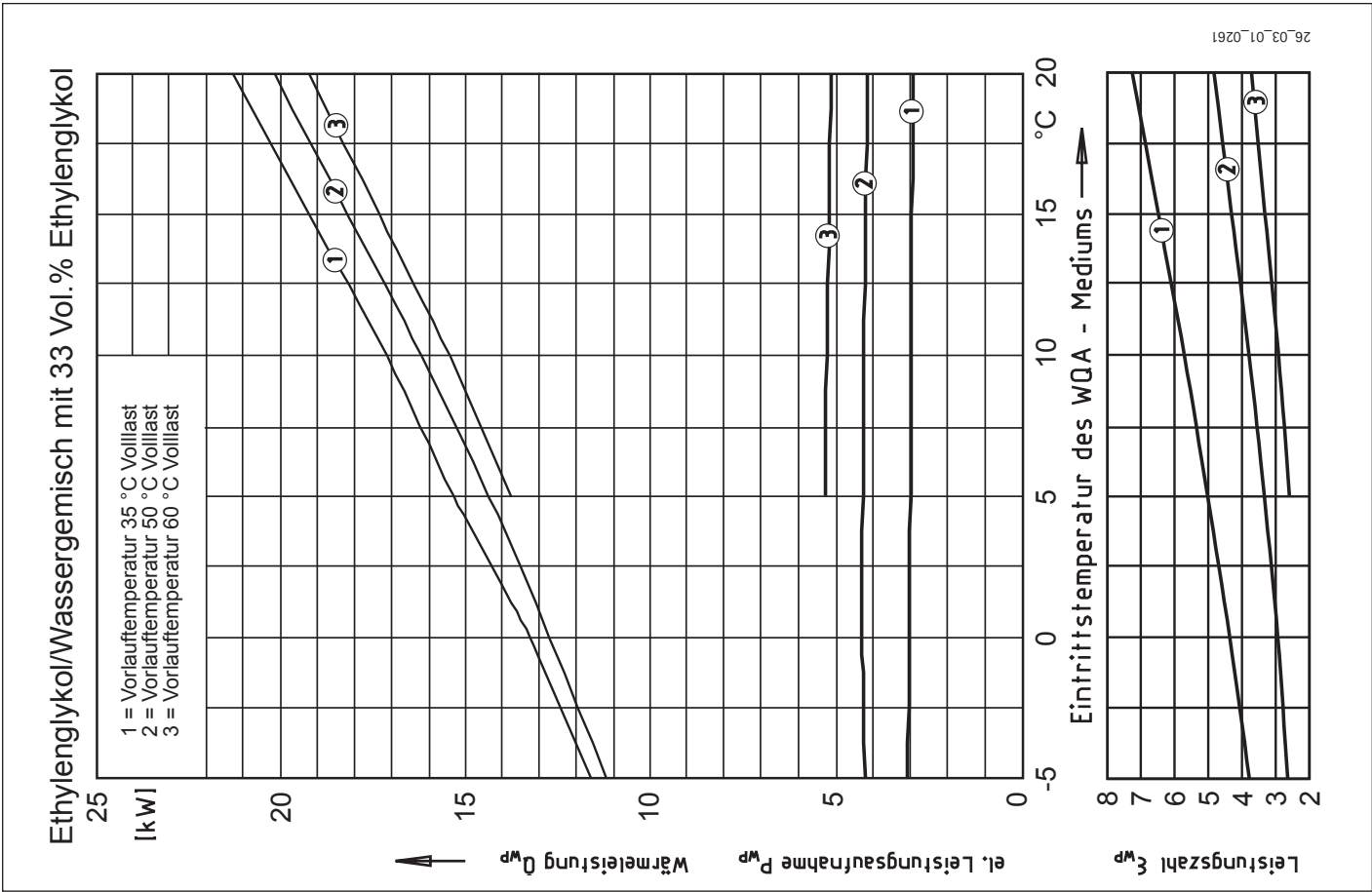
Leistungsdiagramm TTF 13
