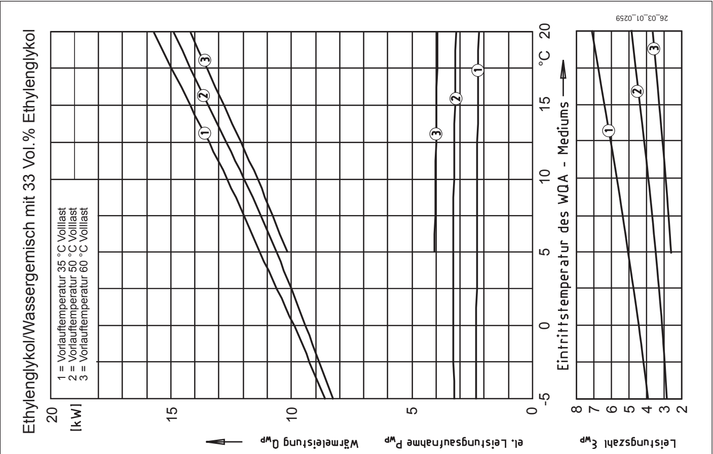
Leistungsdiagramm TTF 10
