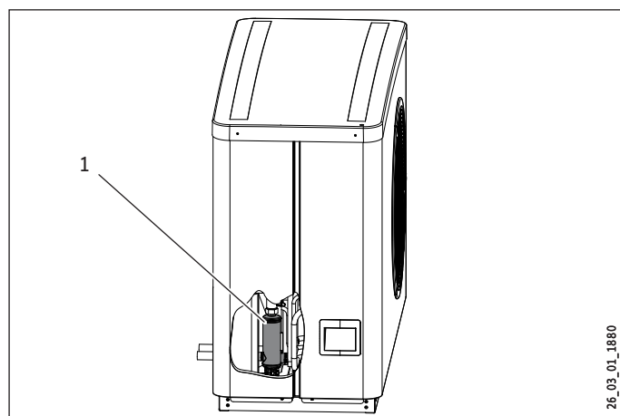
1 Elektrische Not-/Zusatzheizung
