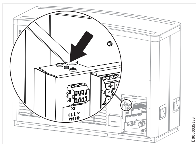
1 Elektrische Not-/Zusatzheizung
