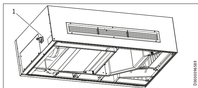
1 Hlavní vypínač
